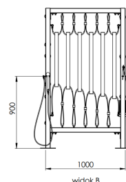
widok B
