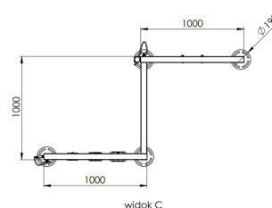
widok C
