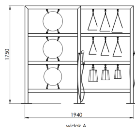
widok A
